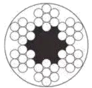
6X7+FC
