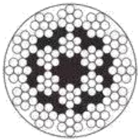
18X7+FC
