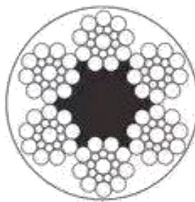
6X19S+FC
