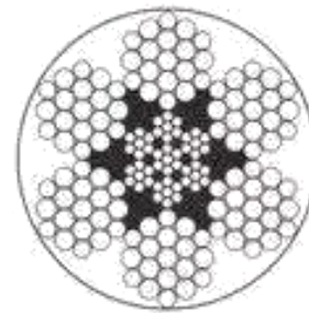
6X19W+IWRC
