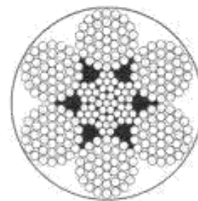
6X37+IWRC
