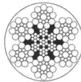
6X19S+IWRC
