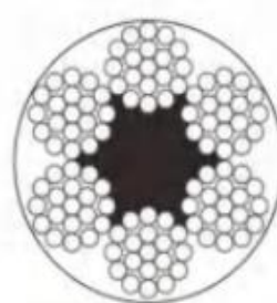
6X19+FC
