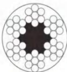
6X7+FC
