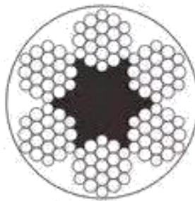
6X19W+FC
