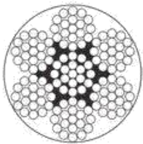
7X19
