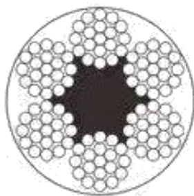
6X19+FC
